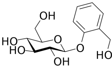
Salicin
