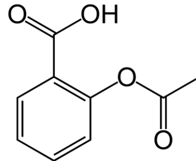
Aspirin
